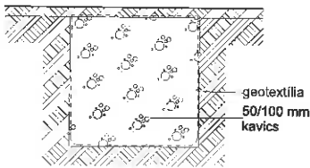
Szikkasztó gödör 2,0 m x 2,0 m x 2,0 m
